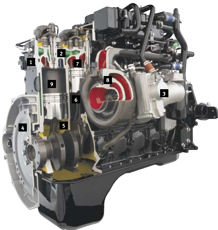
POWERTRAIN/FRAME
