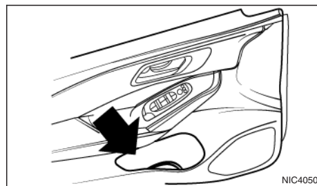
Front door
