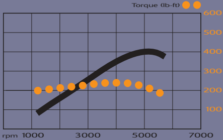
3.8L V6
