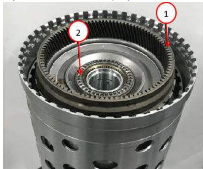
Fig. 29 Input Shaft
